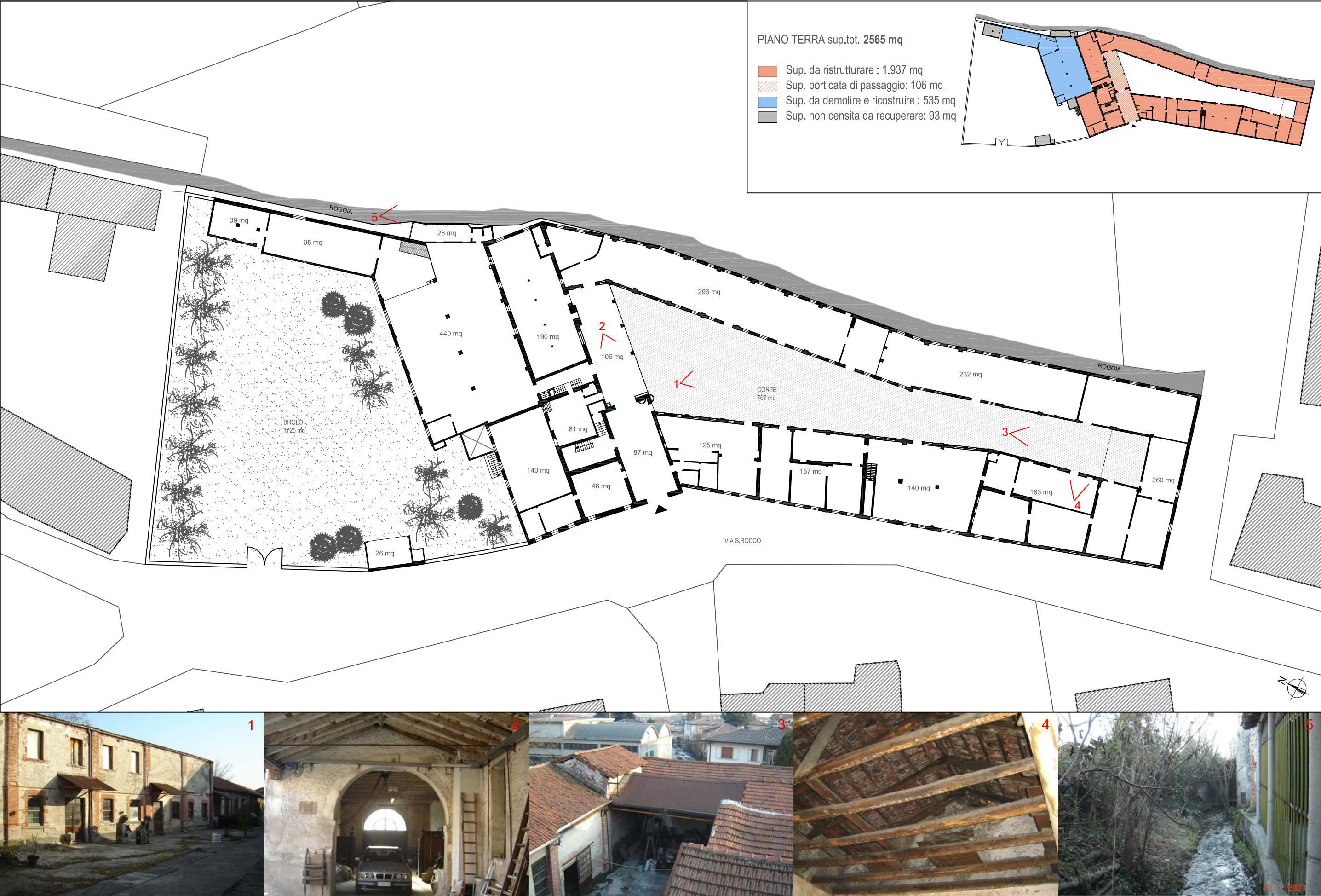
PIANTE PIANO TERRA
